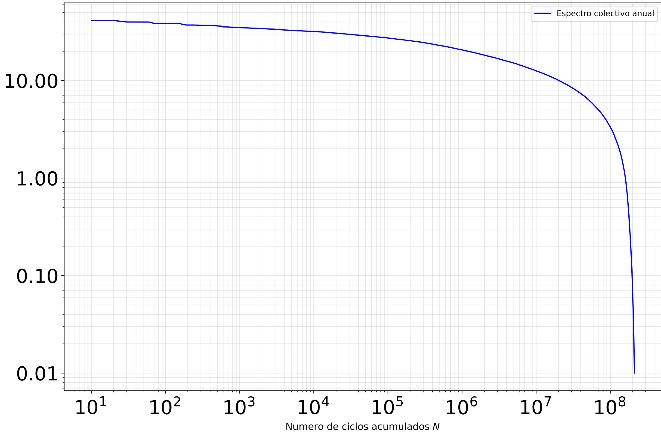
Espectro colectivo anual de fatiga (ponderado Weibull)
